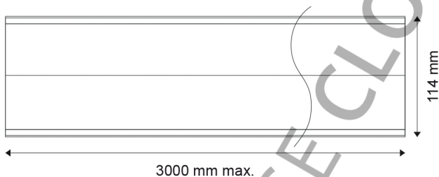
Vue de dessus (éch. : 1/5) :
